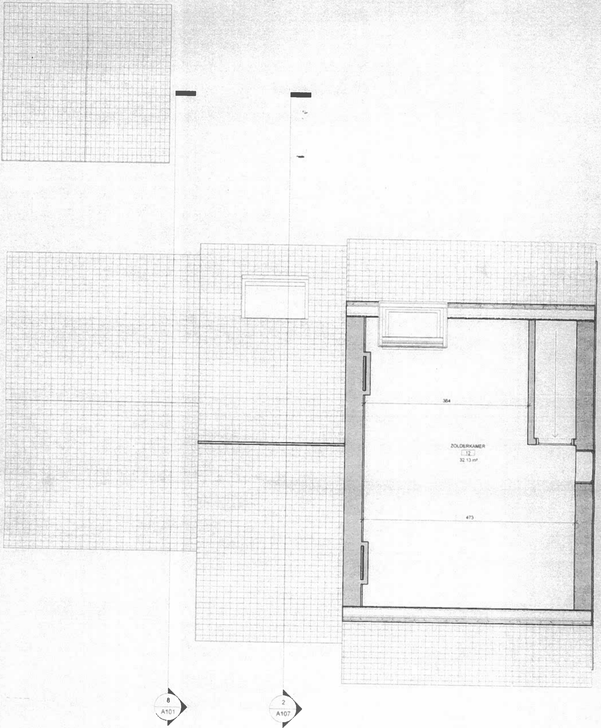
3 20 Tweede Verdieping 1 : 50
