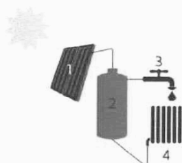
1. Zonnecollector 2. Opslagvat zonnecollectoren 3. Sanitair waterkraan 4. Radiator 5. Warmwaterleiding 6. Warmwaterleiding
