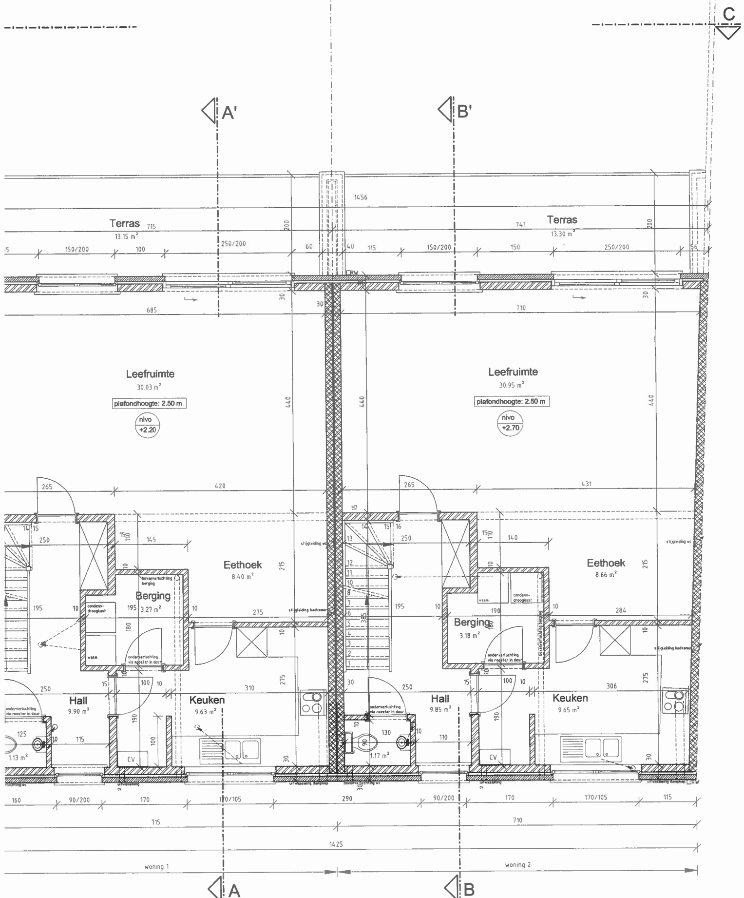
PLAN 1° VERDIEPING
