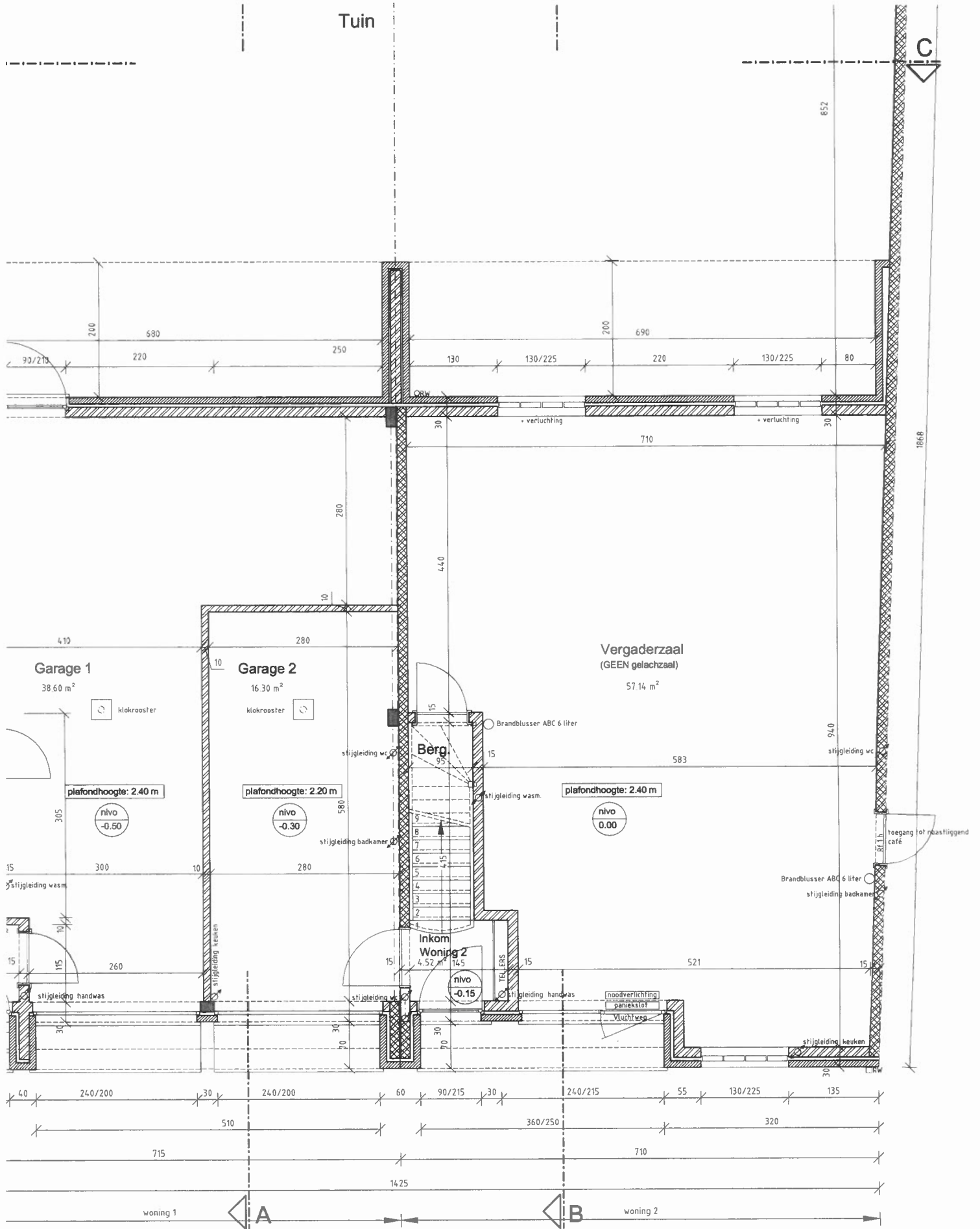
PLAN GELIJKVLOERS
