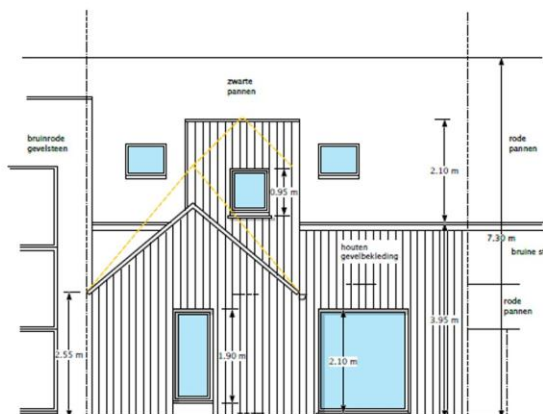
TUINGEVEL - noord (na verbouwing)
