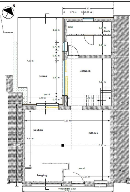
GRONDPLAN (na verbouwing)
