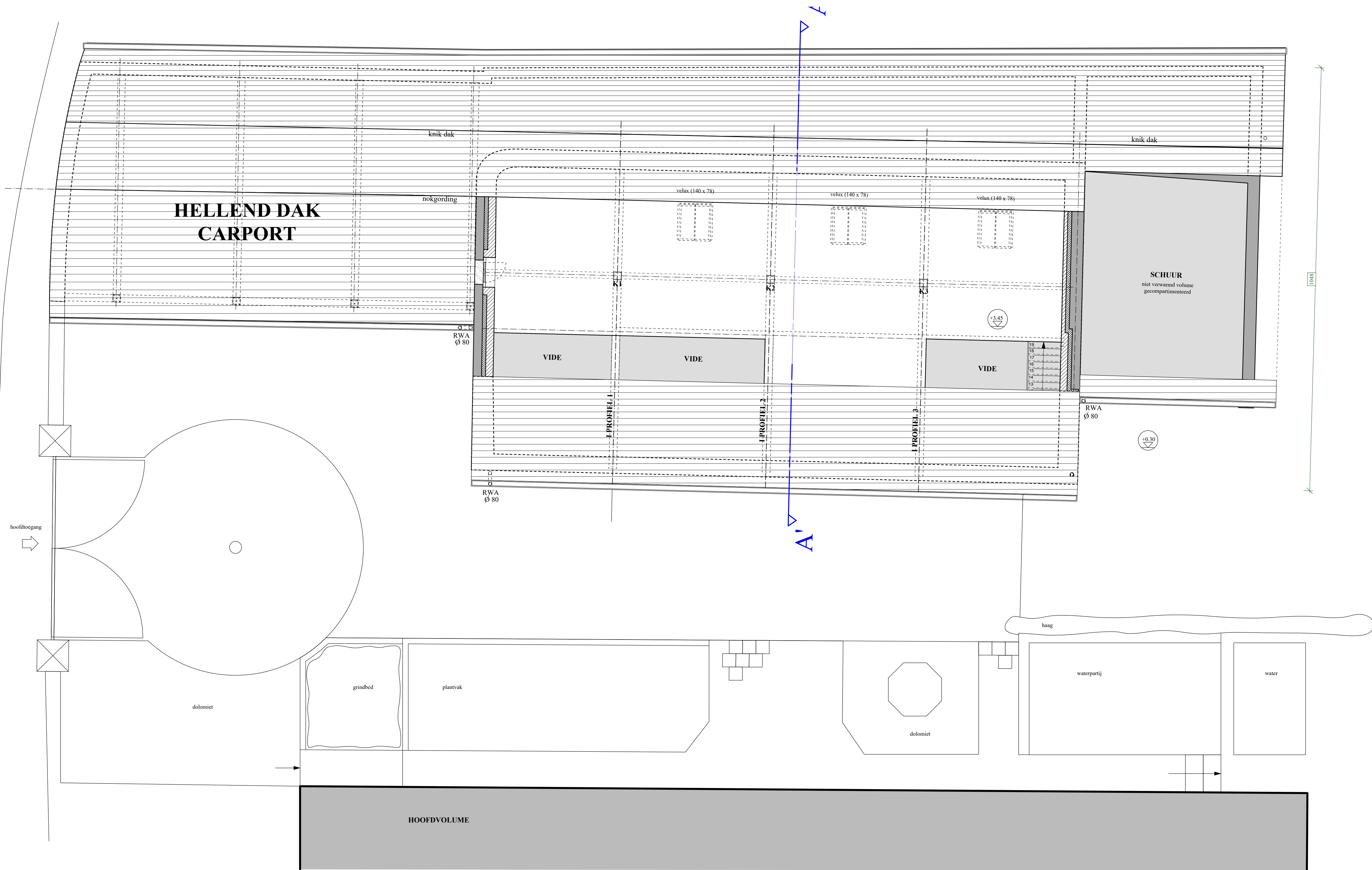
GRONDPLAN VERDIEPING HOBBYRUIMTE Schaal 1:50
