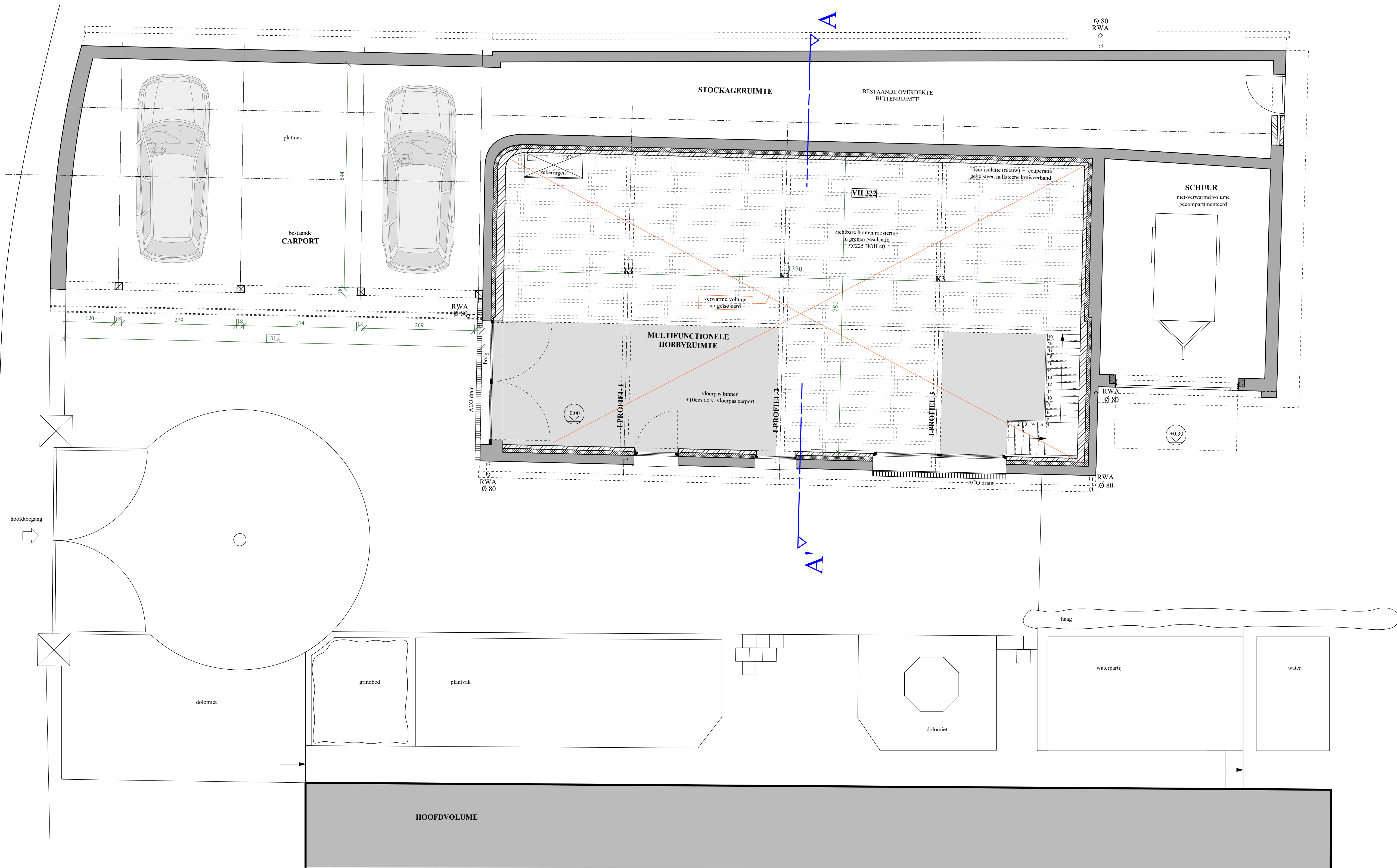
GRONDPLAN GELIJKVLOERS HOBBYRUIMTE Schaal 1:50
