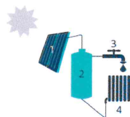
1. Zonnecollector | 2. Opslagvat zonnecollector 3. Sanitair warm water | 4. Afgifteenheid voor ruimteverwarming (voor kiezen)
